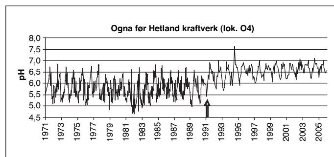
Figur 2.3. Langtidsserier (1971-2005) for pH på stasjon O4 (Hetland, før kraftverket) i Ogna, Rogaland. Data fra effektkontrollen (NINA). Pil angir tidspunkt for når permanent kalking av vassdraget kom i gang.
