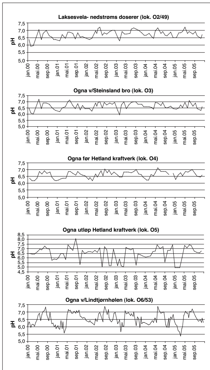
Figur 2.2. pH ved fem stasjoner (O2-O6) i Ogna, Rogaland, i perioden 2000-2005. Data fra effektkontrollen (NINA). Merk: ulik skala på y-aksen.
